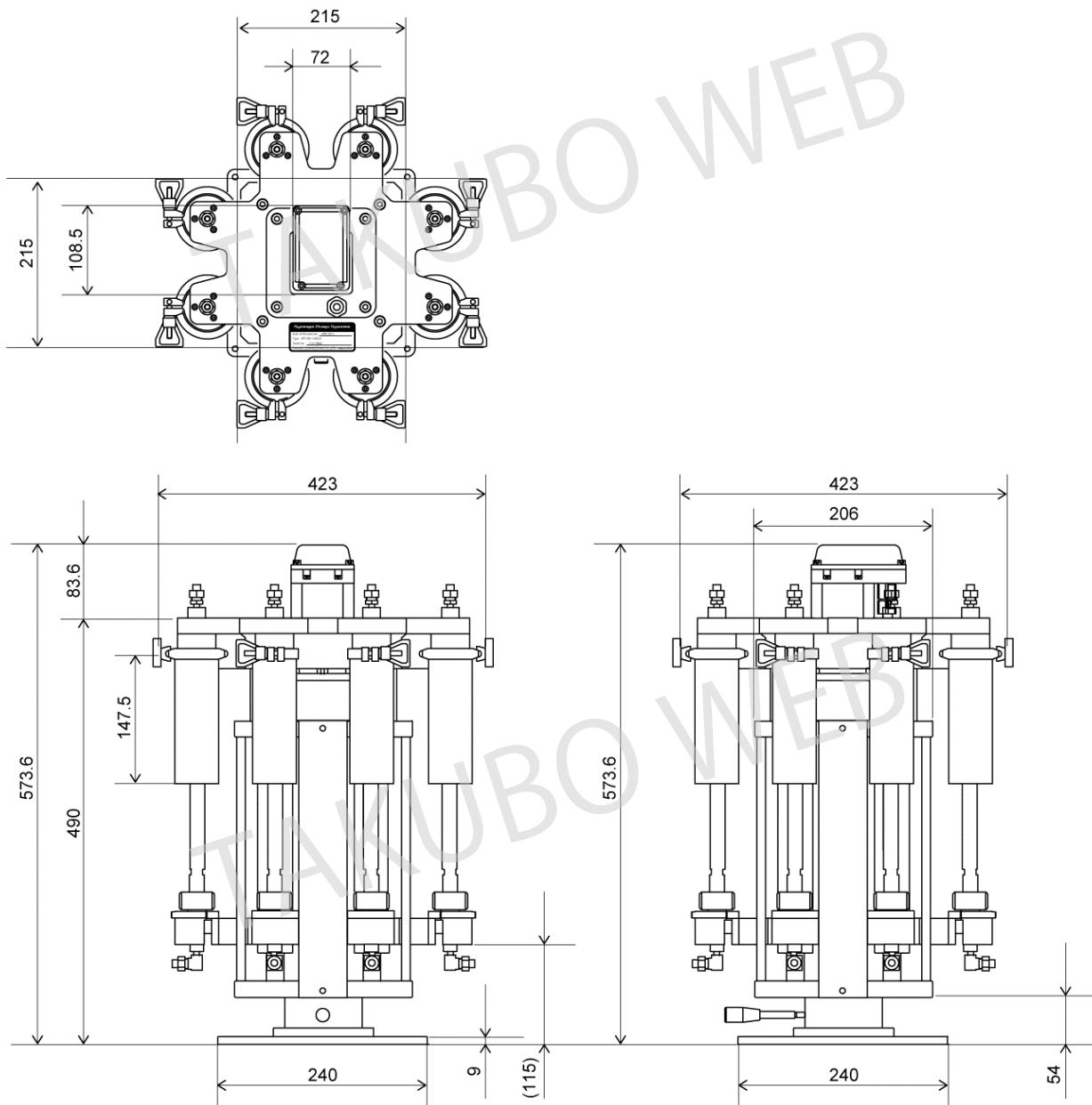
ポンプ本体寸法図
